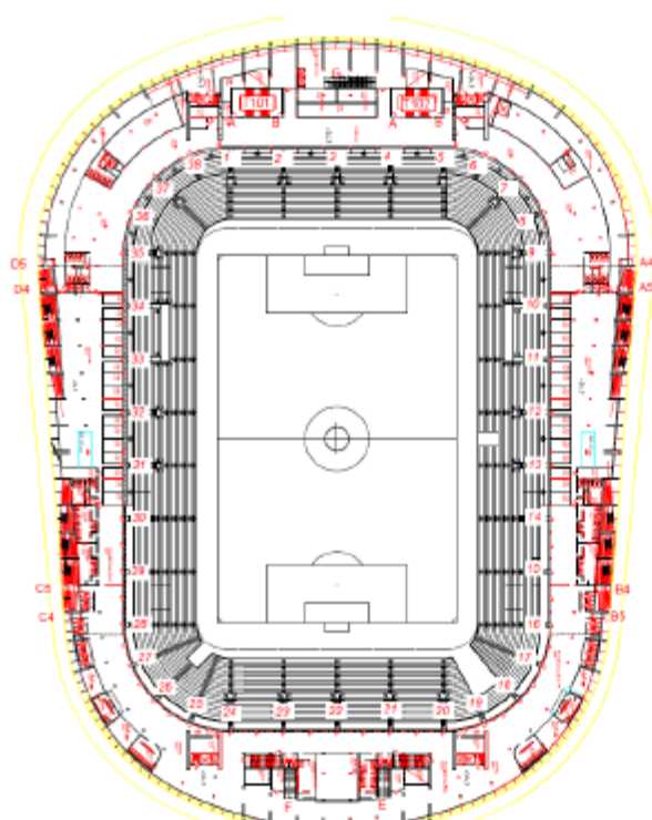
Figur 2.2 Placering samt fria bredder för utrymningsvägar från plan 5.
