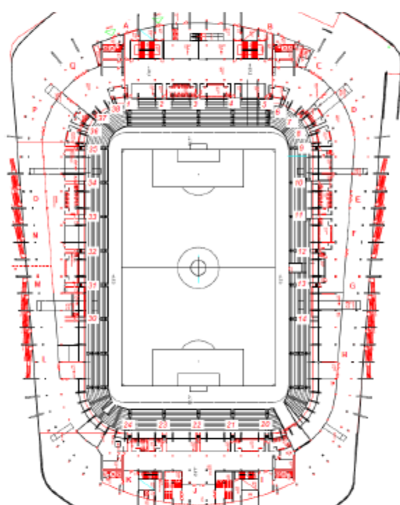
Figur 2.3 Placering samt fria bredder för utrymningsvägar från plan 4.
