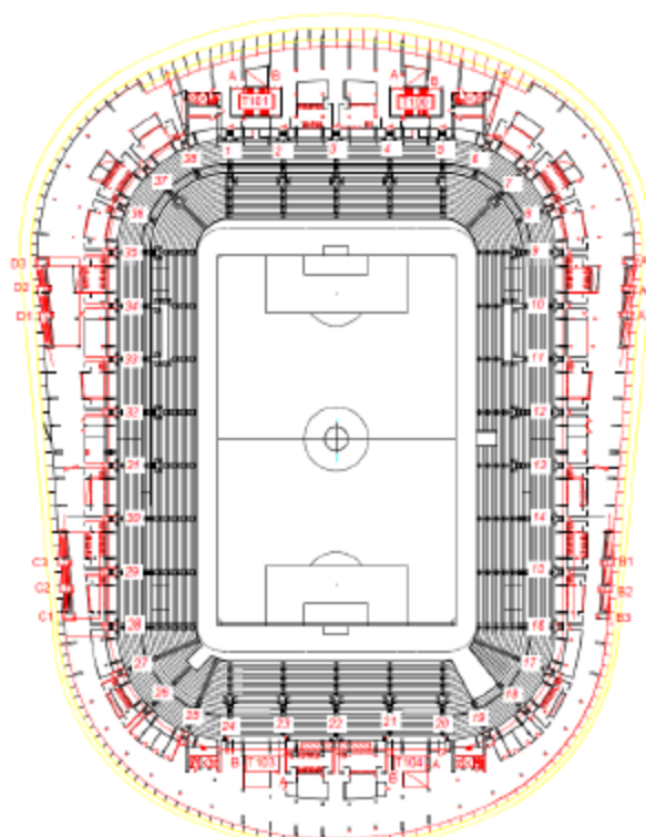
Figur 2.1 Placering samt fria bredder för utrymningsvägar från plan 6.
